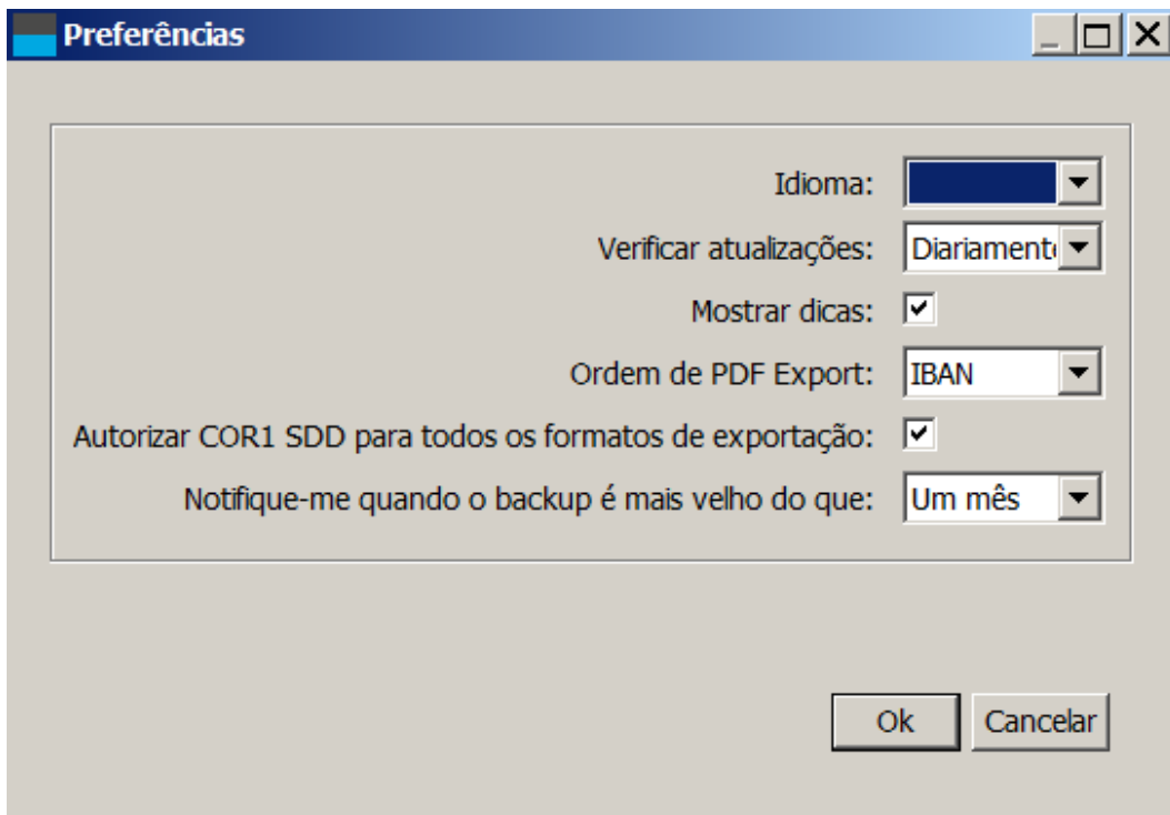
Figura 10: Alterar definições.
