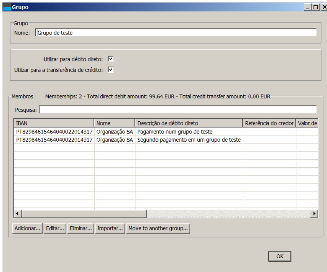
Figura 19: Um grupo que contém a mesma conta duas vezes.
