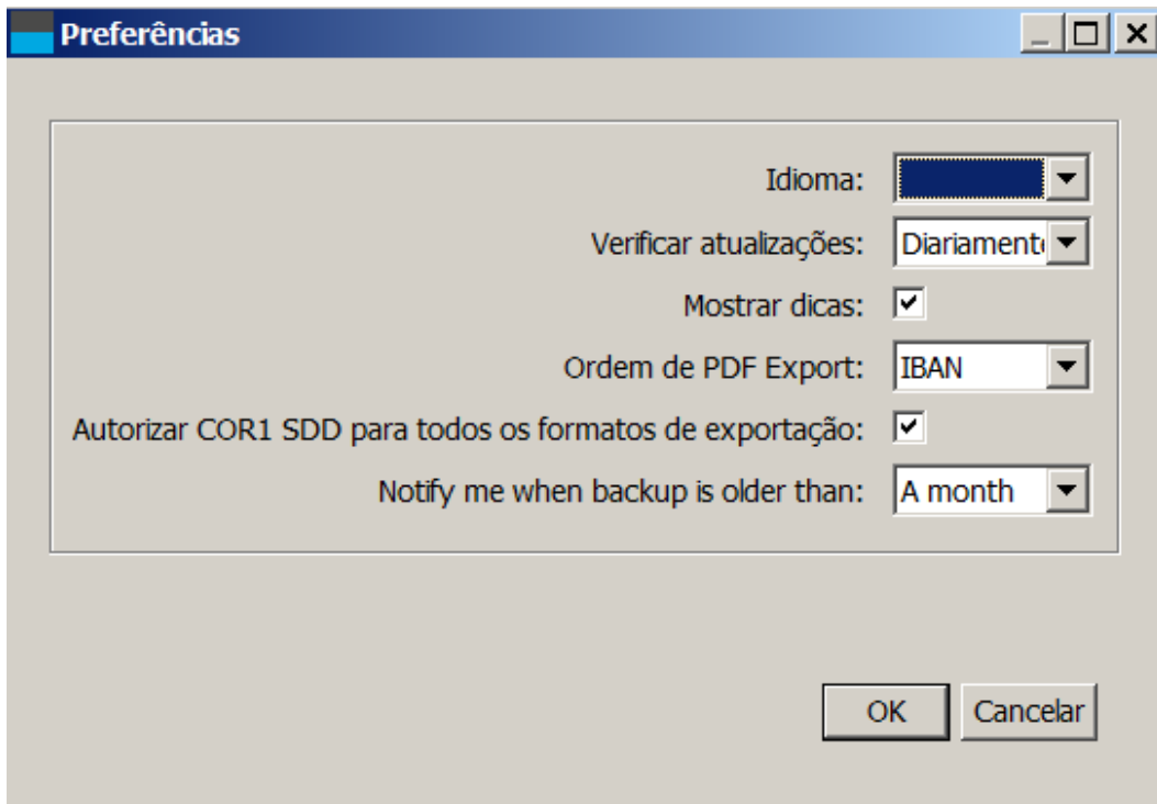
Figura 10: Alterar definições.
